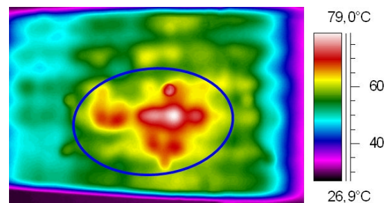
Thermogramm: Hohlstelle (blauer Kreis) in Stahlbetonbauteil
