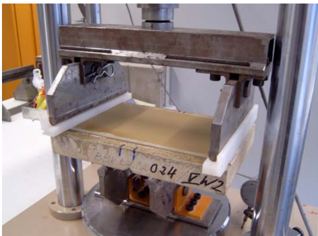
Risserzeugungsversuch
